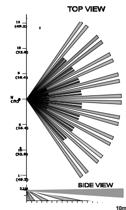
Рис. 5 - Широкоугольная линза
