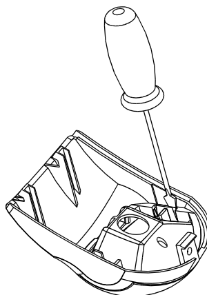
Рис. 6 Замена линзы
