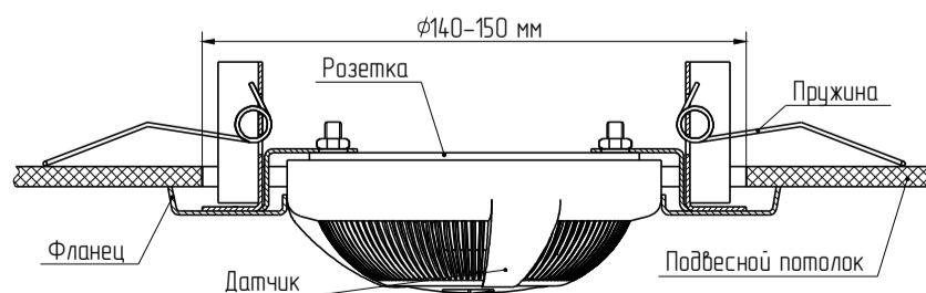
Крепление извещателя к подвесному потолку с помощью пружин и металлического фланца (КМЧ-6)
