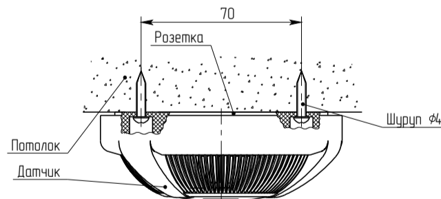
Крепление извещателя к потолку
