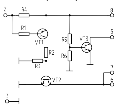
Устройство согласования УС-02. Схема электрическая принципиальная
