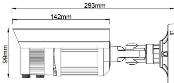
Рис.1 Вид сбоку
