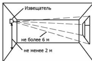
Рис.3. Установка извещателя на противоположной стене
